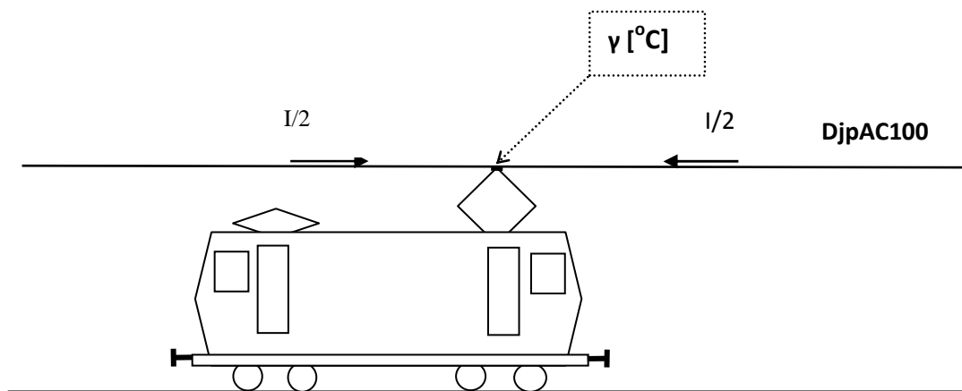
Rys. 2. Szkic stanowiska badawczego w Zakładzie Taboru
