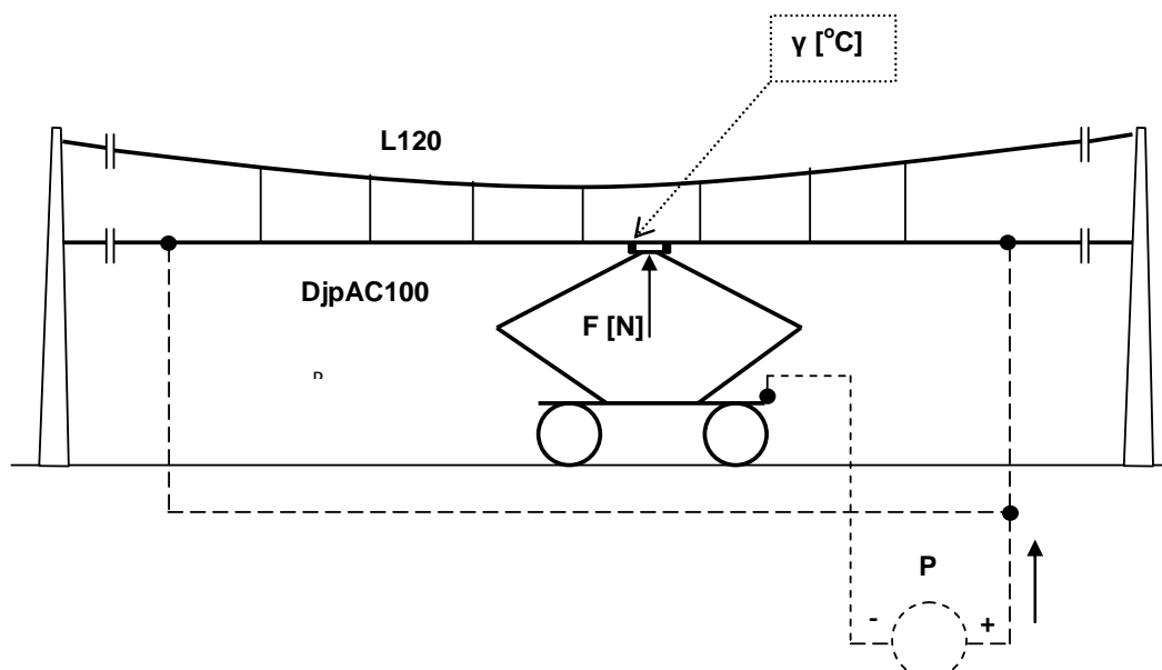
Rys. 1. Laboratoryjne stanowisko badawcze
