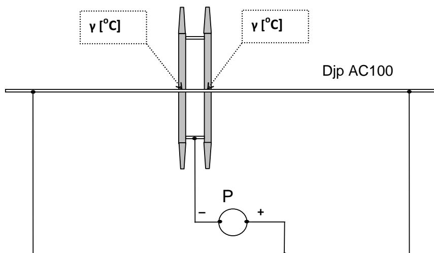
Rys. 3. Punkty pomiaru temperatury przewodu jezdnej
