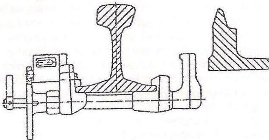
rys. 3 - szczęki mocujące obejmują szynę, a unieruchomiona szczęka ruchoma uniemożliwia dosunięcie iglicy (odsuniętej) odlegającej
