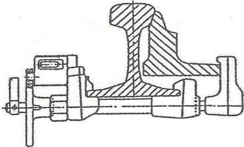
rys. 4 - szczęki mocujące obejmują szynę, a unieruchomiona szczęka ruchoma uniemożliwia odsunięcie iglicy przylegającej
